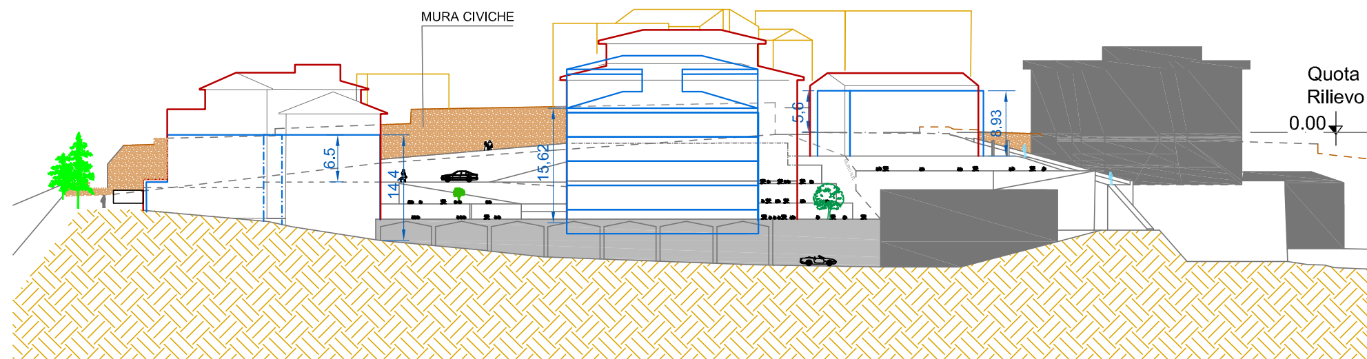
PROSPETTO SUD-OVEST
